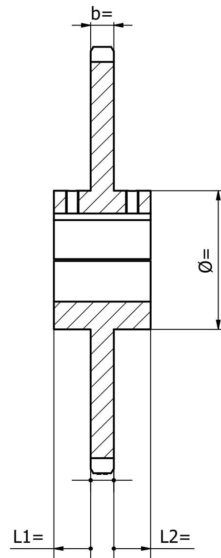
A-A ( 1 : 4 )
